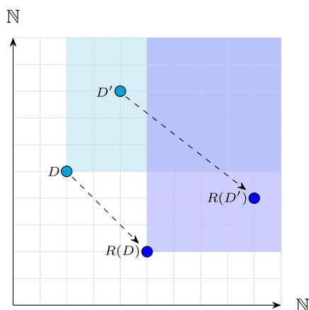
Fig. 2 Visual representation of Lemma 7
