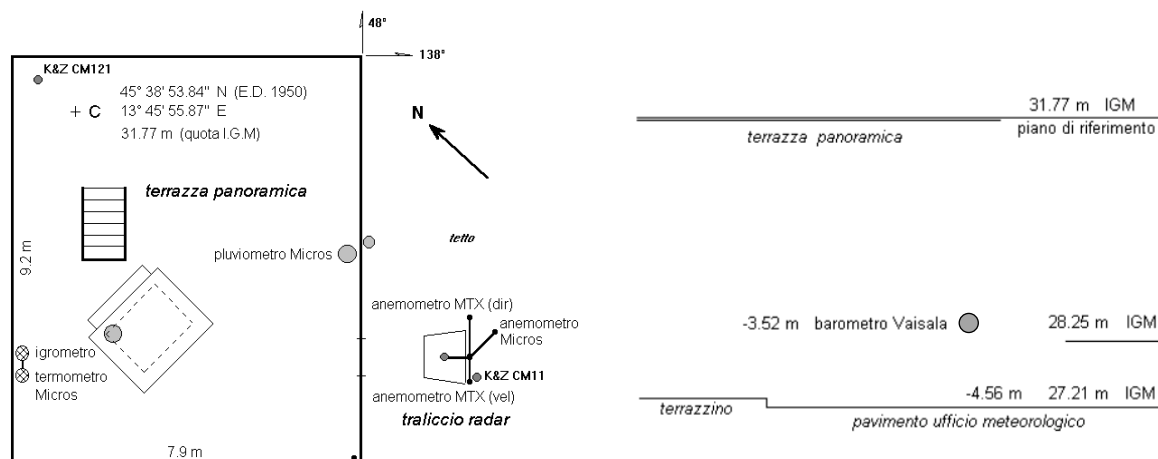
Fig. 1 - Pianta della terrazza panoramica sul tetto dell'I.S.I.S. Nautico e posizione dei sensori meteorologici e del caposaldo C (a sinistra); quota IGM del caposaldo e quote del barometro e del pavimento riferite al caposaldo e allo zero IGM (a destra).
