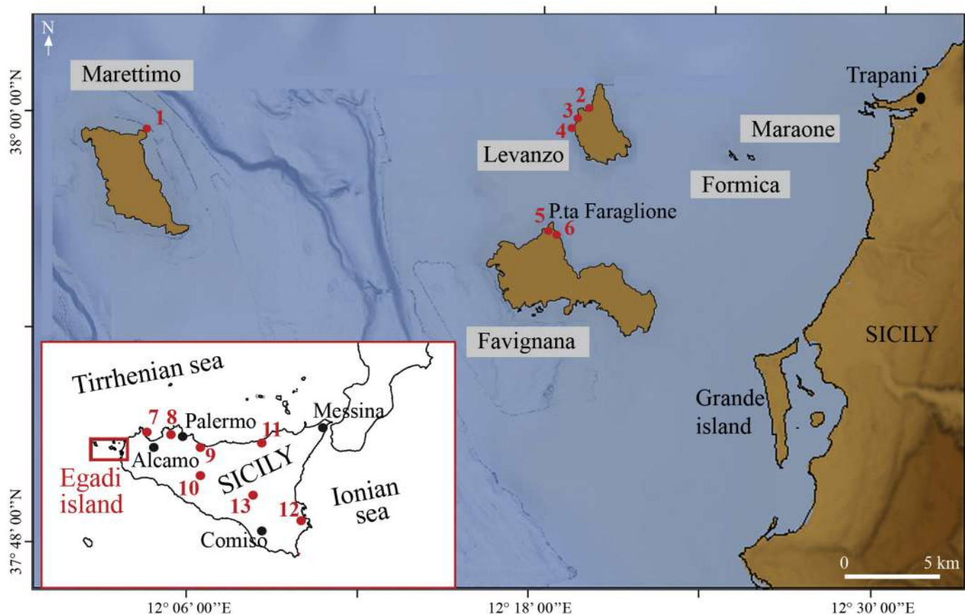
Fig. 1. Egadi Archipelago, geographical setting. 1) Grotta del Tuono, 2) Grotta di Punta Capperi, 3) Grotta Schiacciata, 4) Grotta del Genovese, 5) Grotte di Punta Faraglione, 6) Grotta d'Oriente, 7) Grotta dell'Uzzo, 8) Puntali cave, 9) Riparo del Castello, 10) Acqua Fitusa, 11) San Teodoro (Acquedolci), 12) Spinagallo and 13) Luparello cave.
